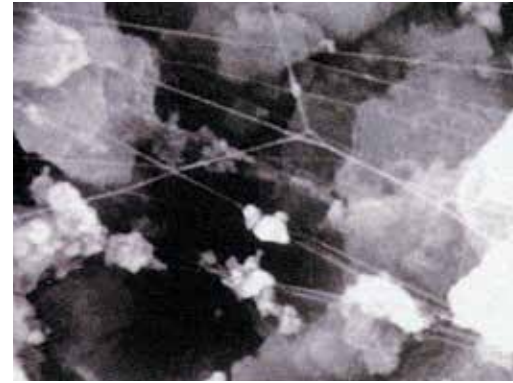
ナイダスト ® の顕微鏡写真 サブミクロン径のテフロン ® 繊維がセメント粒子を捕らえ発塵を防止します。
